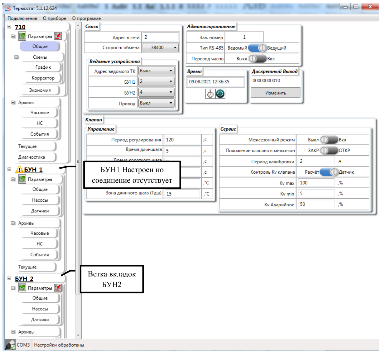
Рисунок 96 – Ошибка подключения одного БУН
