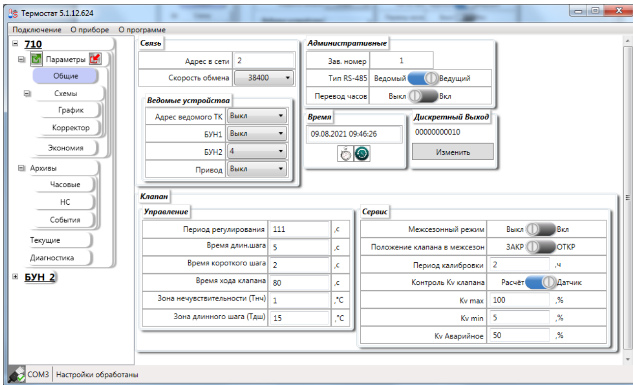
Рисунок 33 –Вкладка «Общие»
