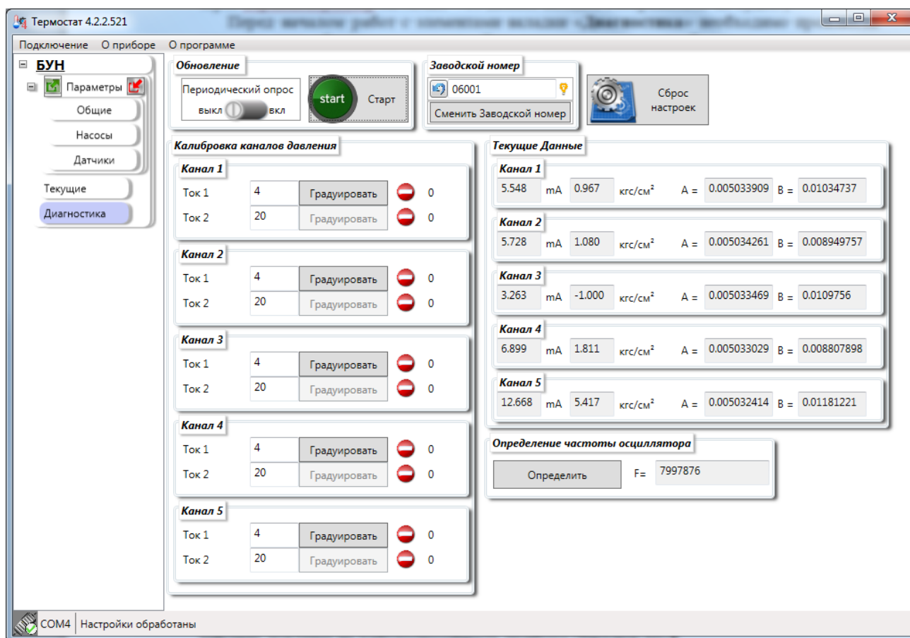
Рисунок 29 – Вкладка «Диагностика»
