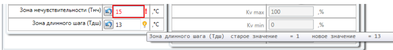
Рисунок 41 – Обработка ограничений
