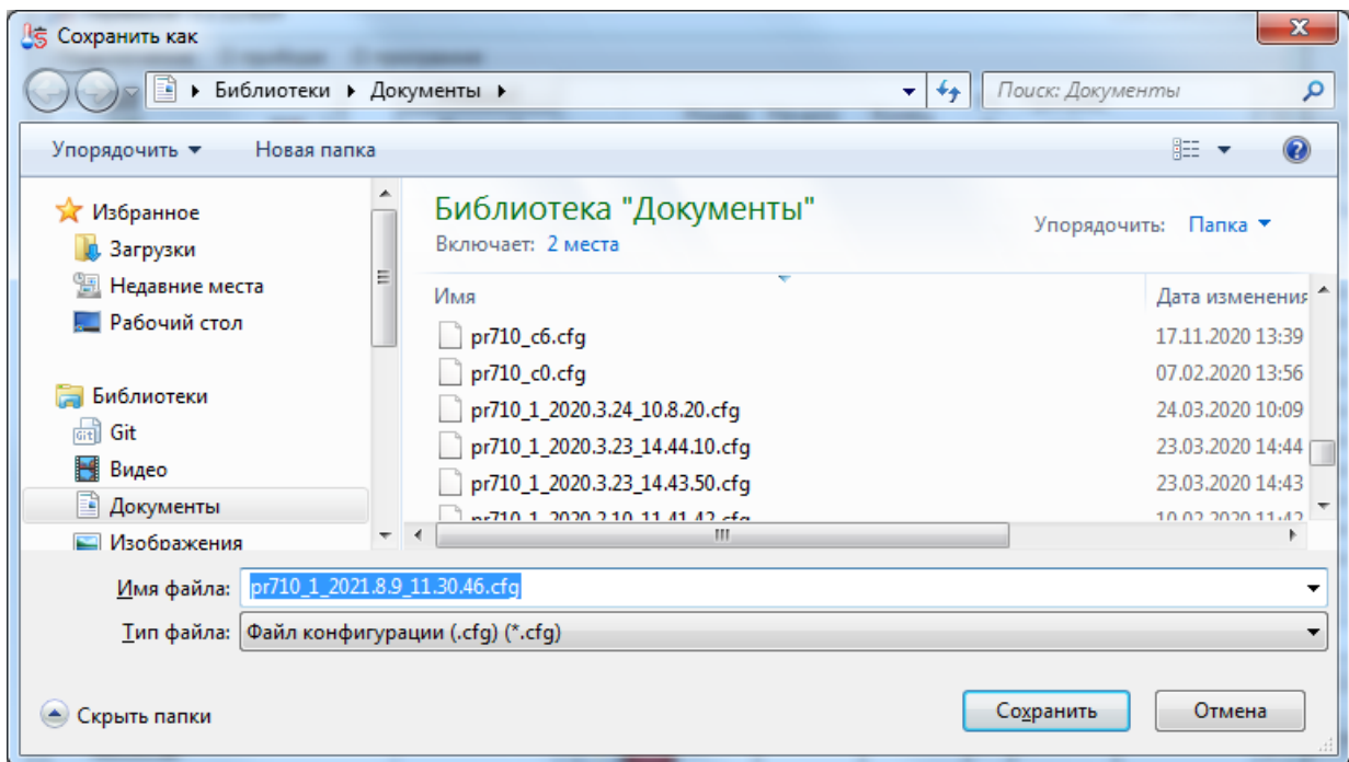
Рисунок 67 – Окно сохранения
